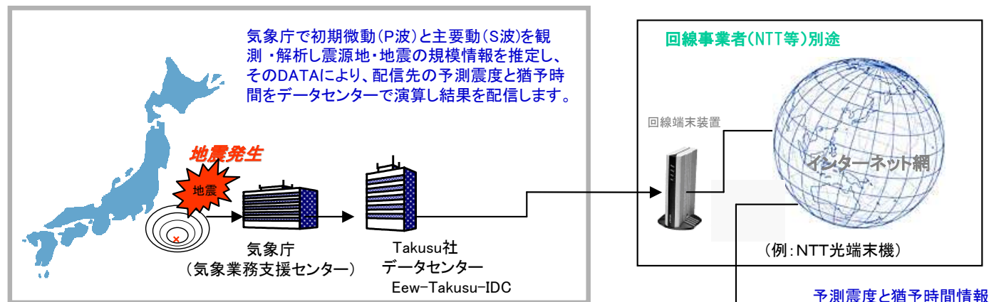
図 1-1 :システム構成図
